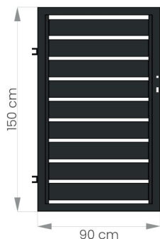
Modern kiskapu:
